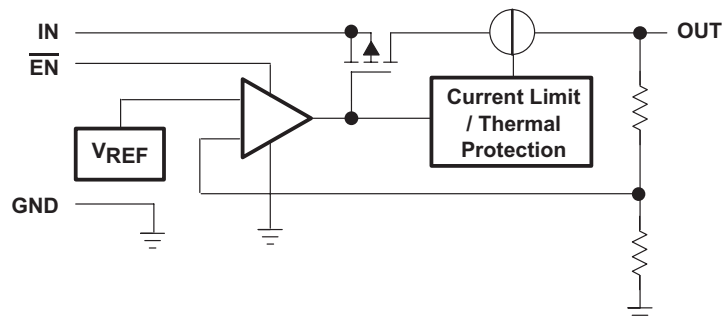
TPS769xx-Q1
