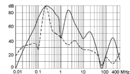
250A (FMAC-0956-H312I)
