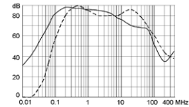
50A (FMAC-0934-5010L)
