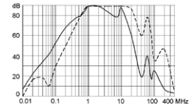
16A (FMAC-0931-1612I)
