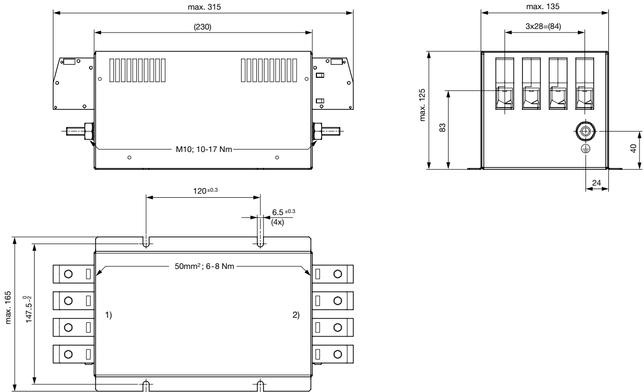
1) Line 2) Load
