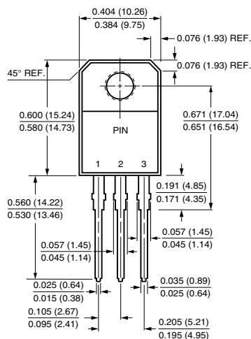
ITO-220AB
